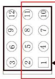
RS485 COM-SW跳帽示意图
