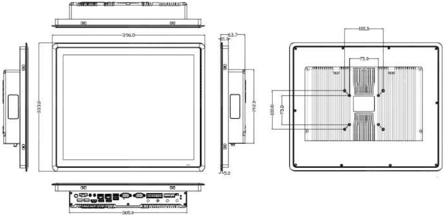
P1771Y-C6 Dimension
