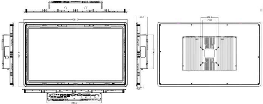
P2381Y-C6 Dimension
